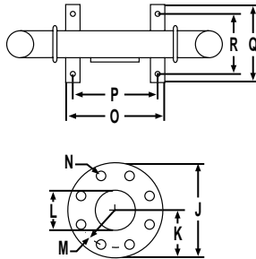
DIMENSIONS - T20 METAL
