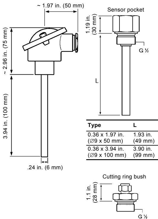
Fig. 70 Dimensions, TTA
