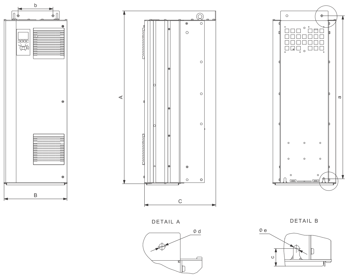
Fig. 52 Enclosures D1h and D2h
