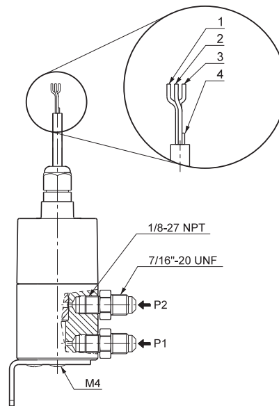
Fig. 69 Wiring diagram, DPI
